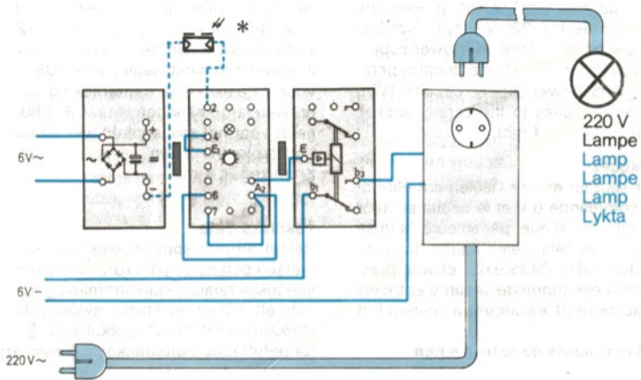
Taktgesteuerte Schaufensterbeleuchtung mit * Sperrung bei Tage, gebaut mit ec 2 oder hobby 4 Fixed cycle control for display window lighting with day-time cut-out, built with ec 2 or hobby 4 Eclairage de vitrine cadencé à interruption diurne, modèle réalisé avec le matériel ec 2 ou hobby 4 Pulsgestuurde etalageverlichting met blokkering bij daglicht, gebouwd met ec 2 of hobby 4 Intervallstyrd skyltffönsterbelysning med fränkoppling på dagen, byggd med ec 2 eller hobby 4
